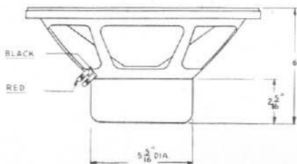
Fig. 1 — Dimensions
